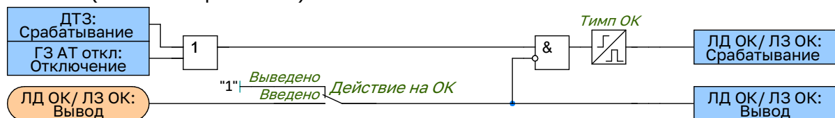
Рисунок 2.39 – Функциональная схема общей логики отключения
