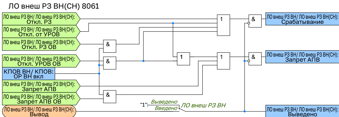
Рисунок 2.35 – Функциональная схема логики внешних отключений ВН
