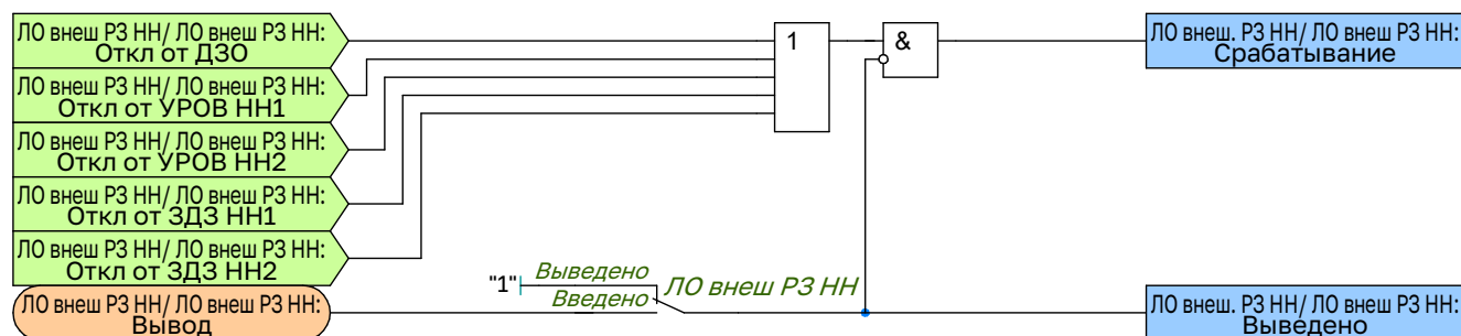
Рисунок 2.37 – Функциональная схема логики внешних отключений НН
