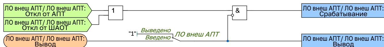
Рисунок 2.38 – Функциональная схема логики внешних отключений АПТ
