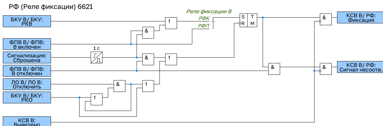
Рисунок 2.34 – Функциональная схема логики реле фиксации выключателя
