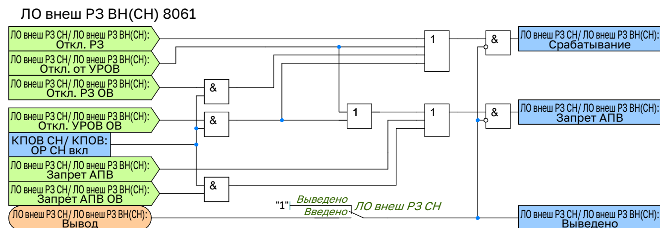
Рисунок 2.36 – Функциональная схема логики внешних отключений СН
